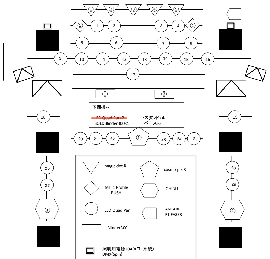
ROXY照明基本仕込図 (2021.6.29現在)
